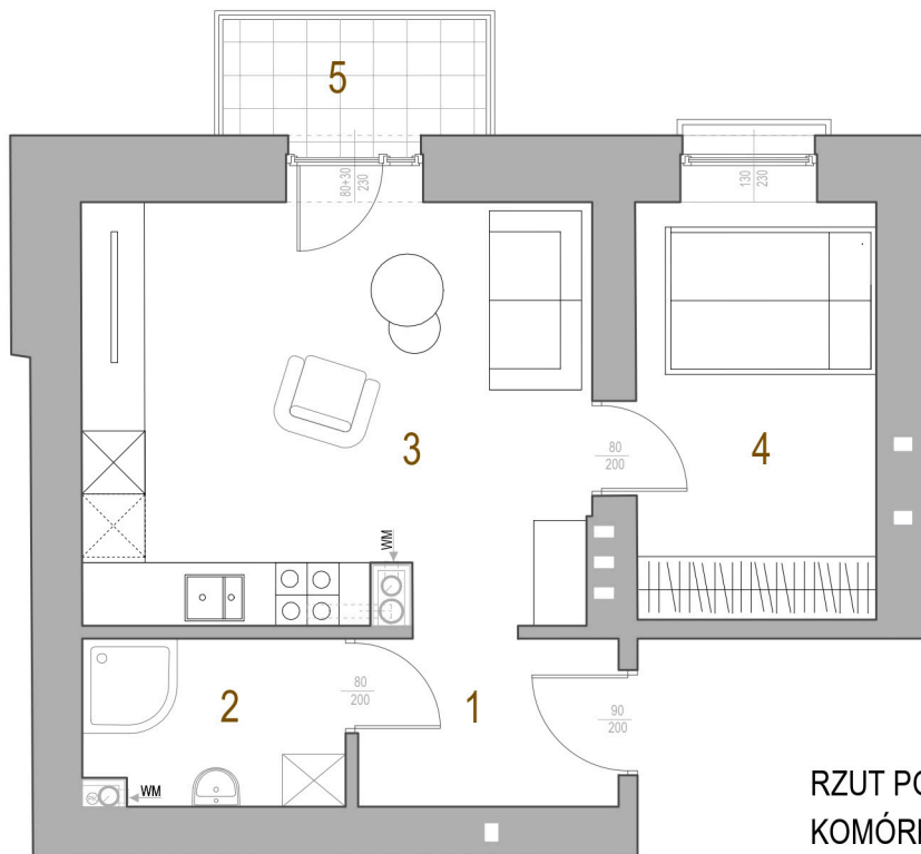
RZUT POZIOMY LOKALU MIESZKALNEGO M6 SEGMENT B
