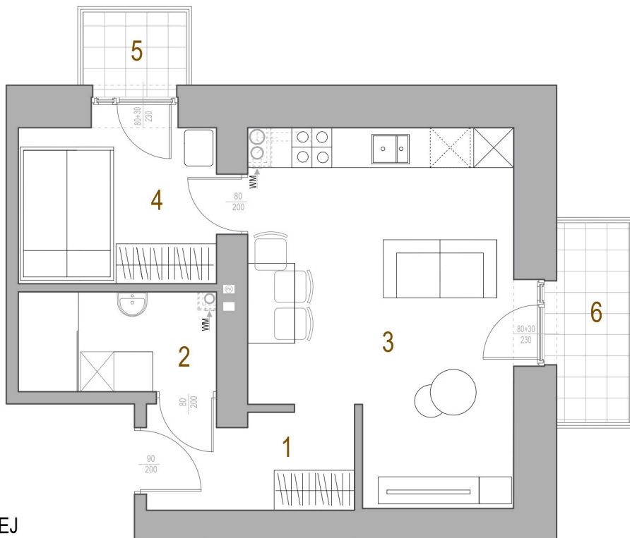
RZUT POZIOMY LOKALU MIESZKALNEGO M3 SEGMENT B
