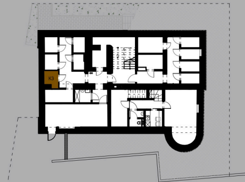
SEGMENT B MIESZKANIE NR 3 2 POKOJOWE 36.22 m 2 RZUT POZIOMY PIWNICY RZUT POZIOMY I PIĘTRA
