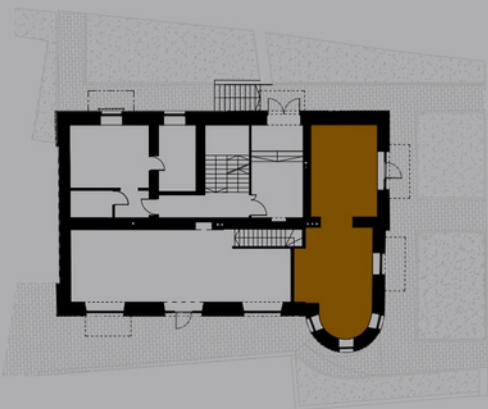
RZUT POZIOMY PARTERU
